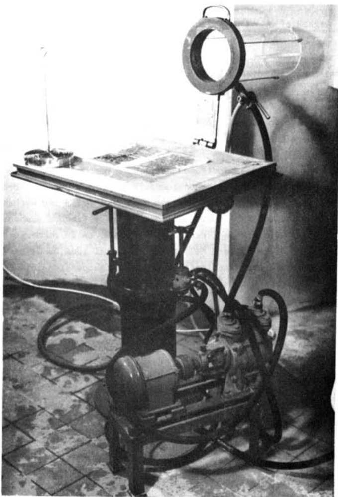
Anfaserungsgerät mit geöffnetem Zylinder, eingelegtem beschädigtem Blatt. Absaugvorrichtung darunter. Auf dem Gitterrahmen links Gerät zum Niederhalten des beschädigten Blattes während des Aufwirbelns der Fasersuspension im Zylinder. Restaurieranstalt der Niederösterreichischen Landesbibliothek.
